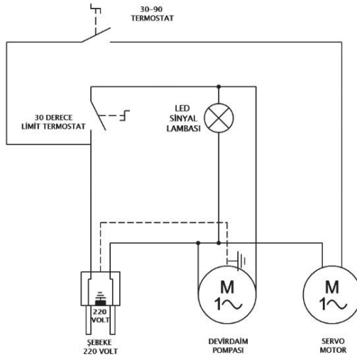
Şekil 5 – EKO SK-25 Servo Motorlu Kumanda Paneli
