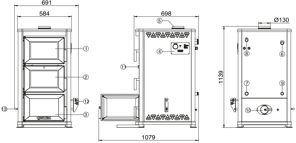
Şekil 1 – EKO SK-25 Soba Genel Görünüşü
