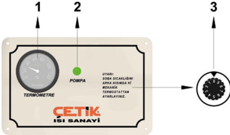
Resim 1 – EKO SK-25 Mekanik Termostat Kumanda Paneli
