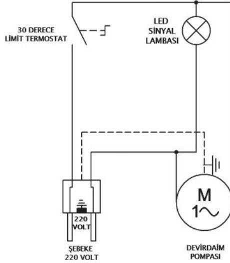
Şekil 4 – EKO SK-25 Mekanik Termostat (Servosuz) Kumanda Paneli
