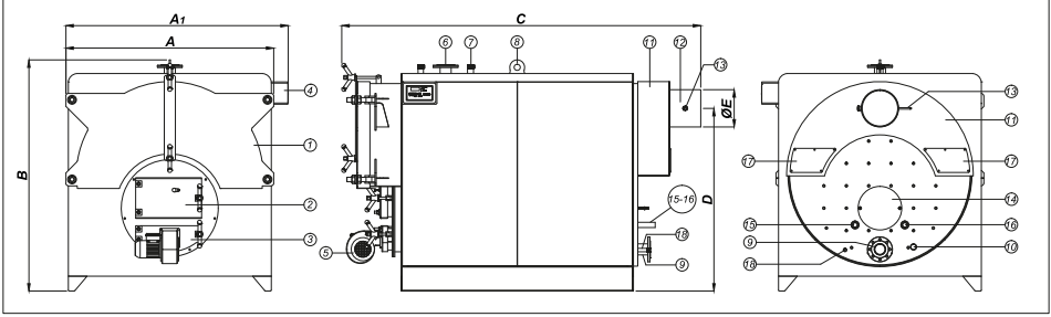
Şekil 1 – Kazan Genel Görünüşü EKO UB-150-...-1500
