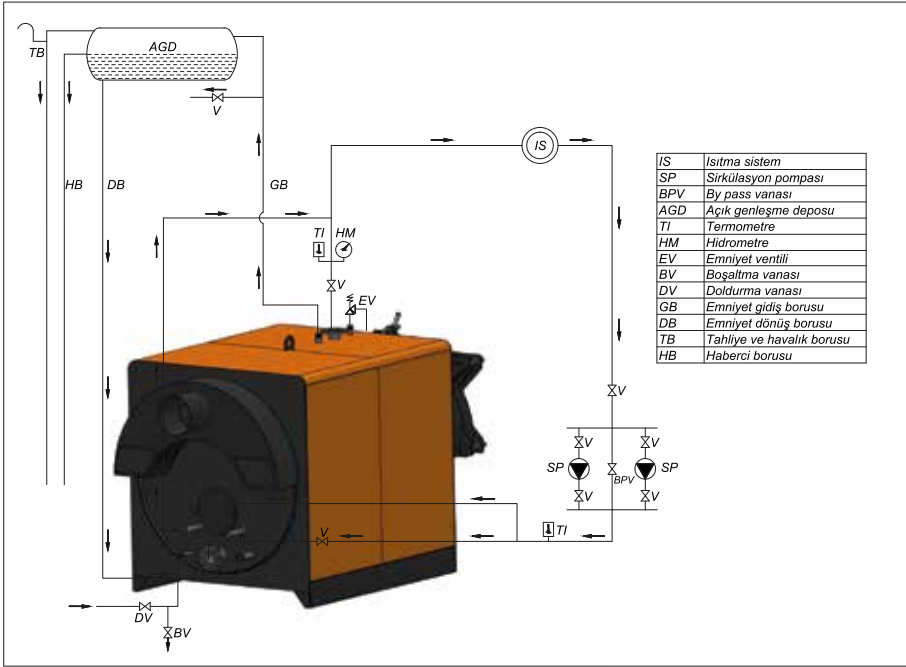
Şekil 2– Tesisat Şeması EKO UB-150-...-1500
