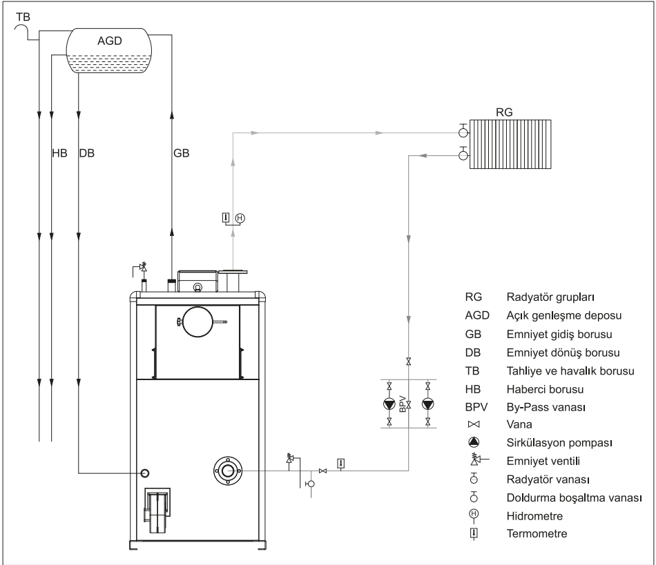
Şekil 4 – Tesisat Şeması EKO B-100...-200
