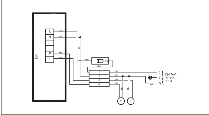
Şekil 8 – EKO B-20-...-80 Elektrik Bağlantı Şeması ( Dijital Kumanda Paneli )
