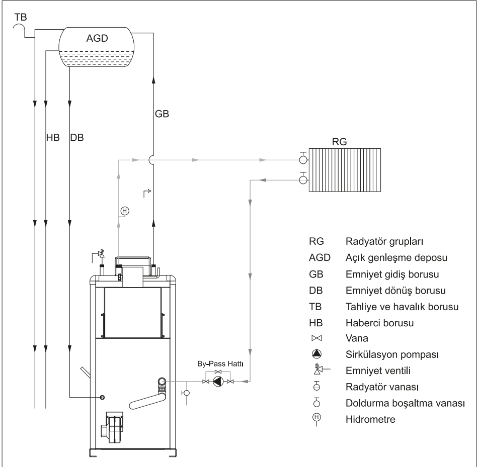
Şekil 3 – Tesisat Şeması EKO B-20...-80
