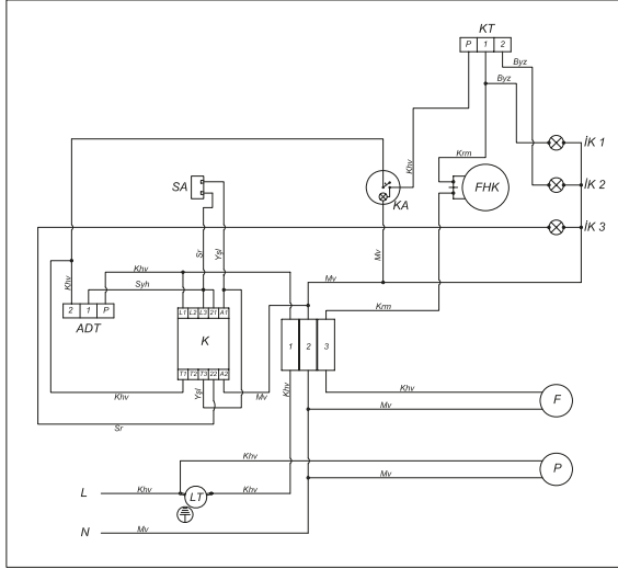
Şekil 6 – EKO B-20-...-80 Elektrik Bağlantı Şeması
