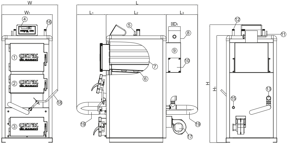
Şekil 1 – EKO B - 20-...-80 Kazan Genel Görünüşü
