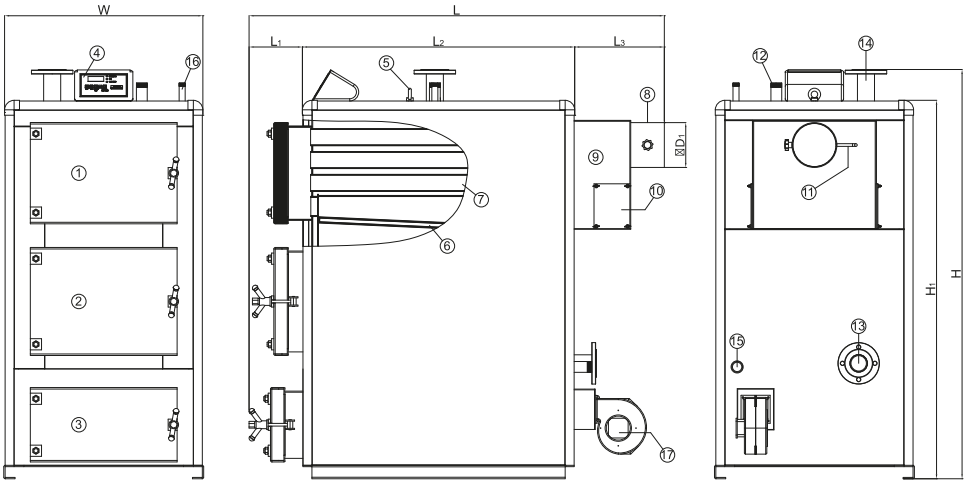
Şekil 2 – EKO B- 100-...-200 Kazan Genel Görünüşü
