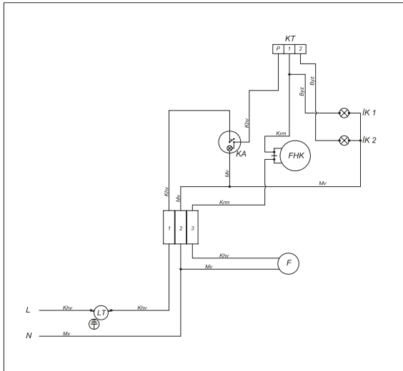
Şekil 7 – EKO B-100-...-200 Elektrik Bağlantı Şeması
