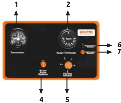
Resim 2 – EKO B-100-...-200 Kumanda Paneli
