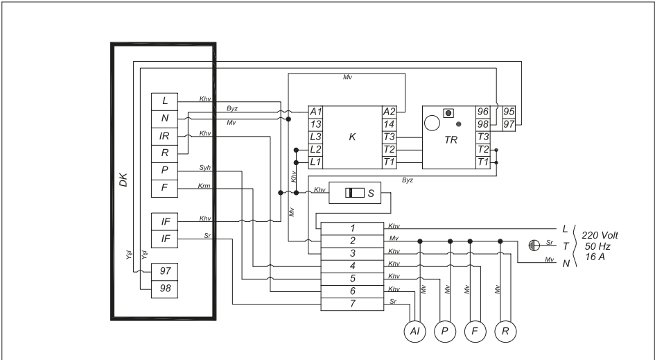
Şekil 7 – EKO BS-20-...-80 Elektrik Bağlantı Şeması Otomatik Tutuşturuculu
