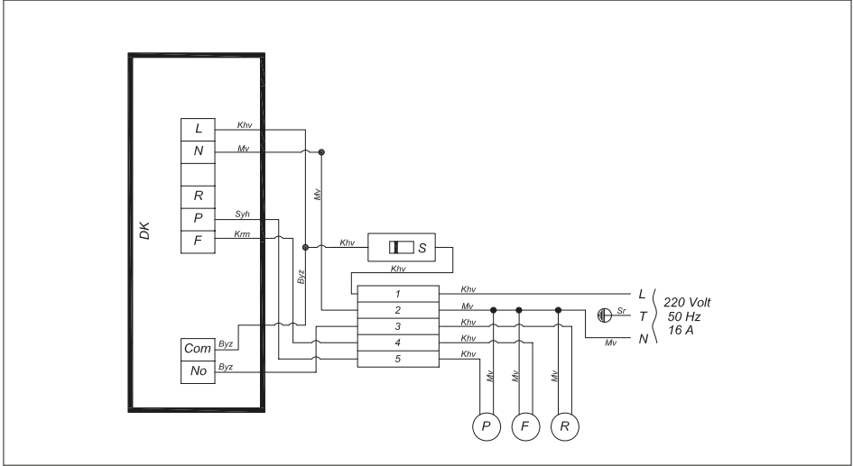
Şekil 6 – EKO BS-20-...-80 Elektrik Bağlantı Şeması
