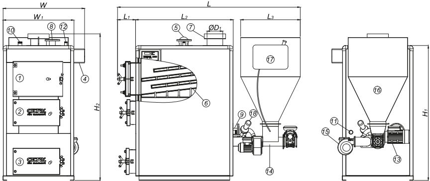
Şekil 2 – EKO S 120-...-300 Kazan Genel Görünüşü
